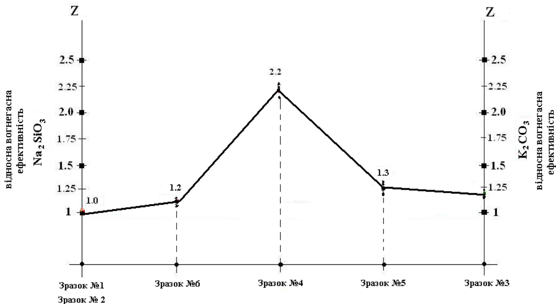
Рисунок 2 - графік залежності відносної вогнегасної ефективності при гасінні нестандартного модельного вогнища класу А в залежності від пропорційного вмісту рідкого натрієвого скла – \text{Na}_2\text{SiO}_3 та карбонату калію - \text{K}_2\text{CO}_3 .
