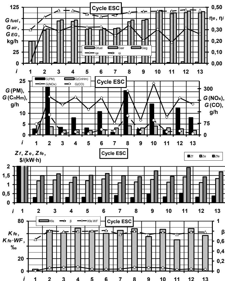
Рис. 1. – Розподіл значень техніко-економічних, екологічних показників роботи дизеля 2Ч10,5/12 та критерію K_{fe} і його складових по режимах випробувального циклу ESC
