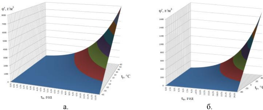
Рис. 1. – Залежність масової концентрації парів бензину Б-70 \Phi' у вертикальному сталюму резервуарі РВС-1000 (а) та РВСП-1000 (б) від часу випаровування \tau_v і температури рідини t_p
