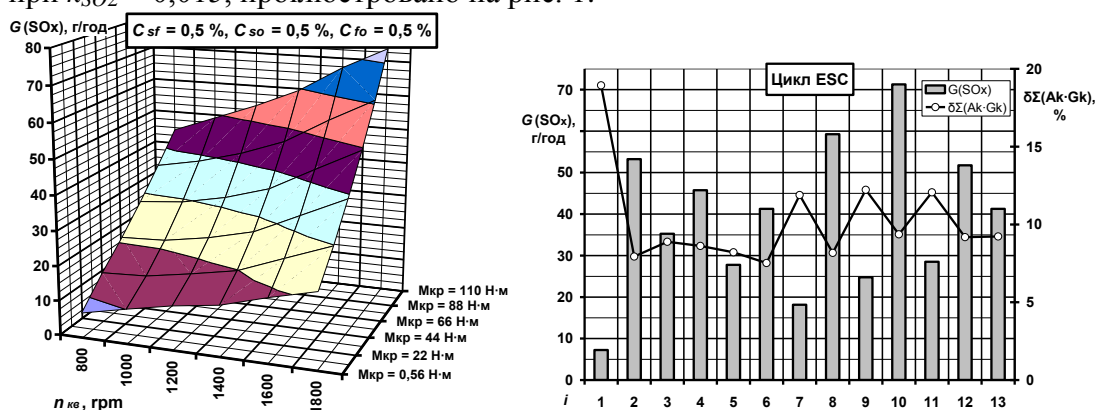
Рис. 1. – Розподіл значень величини G(\text{SO}_x) по режимах стандартизованого стаціонарного випробувального циклу ESC для автотракторного дизеля 2Ч10,5/12
