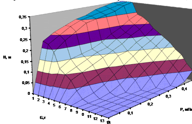
Рис. 1. Залежність висоти підйому вантажу від маси вантажу і тиску повітря в оболонці, для ПР ПТО розміром 0,5 \times 0,5 м
